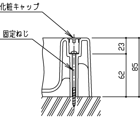
固定部詳細(尺度フリー)
